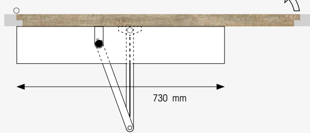
Normalgestänge | drückend | Sturzmontage
